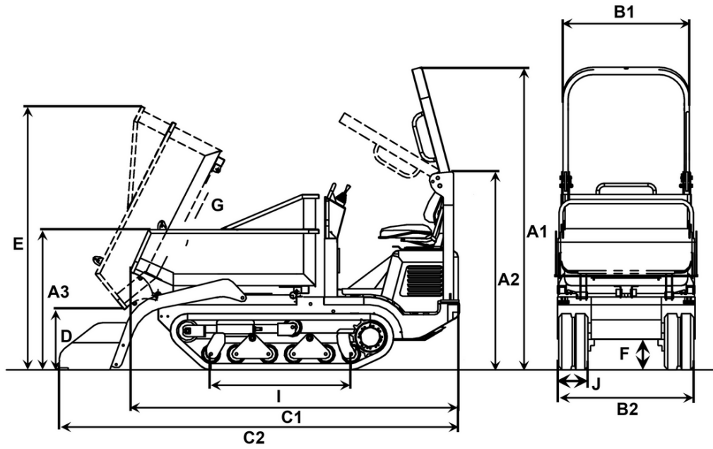
Tolva frontal/Volquete giratorio/Tolva en altura/Plataforma basculante de 3 lados/Hormigonera
