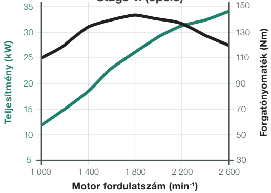
Teljesítménygörbe Yanmar 3TNV86CHT; 33,3 kW; Stage V. (opció)
