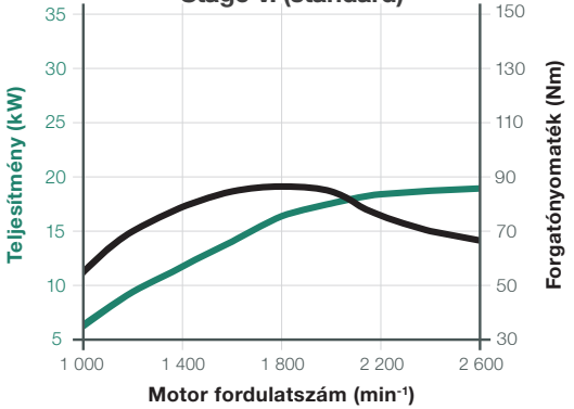
Teljesítménygörbe Yanmar 8TNV80FT; 18,4 kW; Stage V. (standard)
