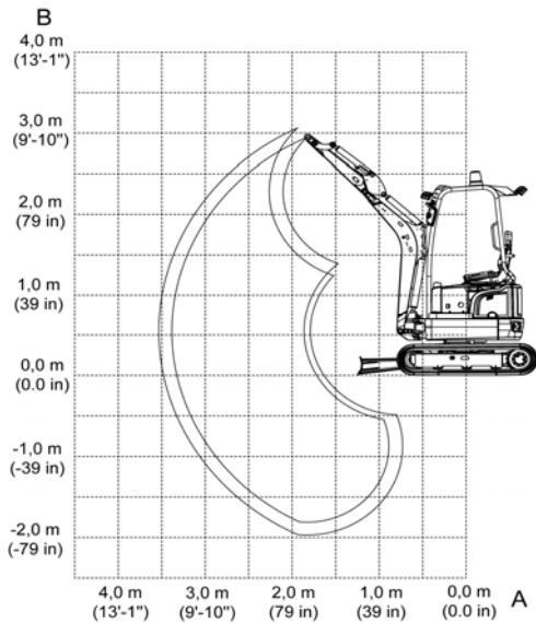
Abb.1: Hubkrafttabelle EZ17
