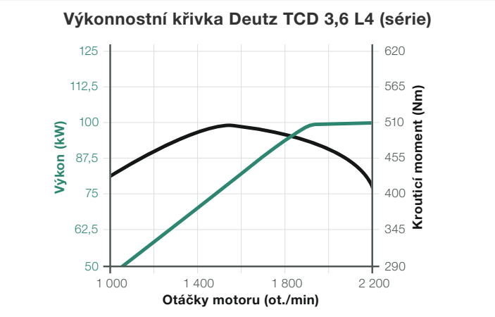
Vodou chlazený čtyřválcový řadový motor s recirkulací výfukových plynů, turbodmychadlem a mezichladičem.
