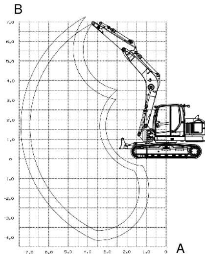
Abb. 1: Hubkrafttabelle 14504
