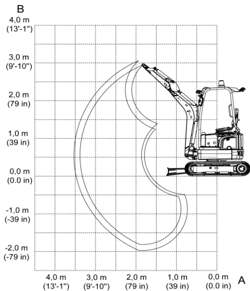
Abb.1: Hubkrafttabelle EZ17e
